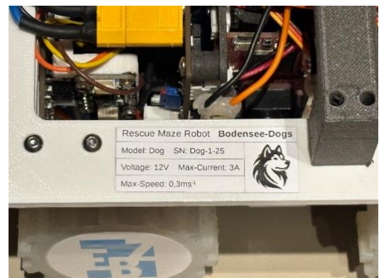
Typenschild des Roboters
